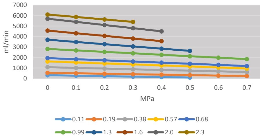
DDS-ELDHD性能曲線
