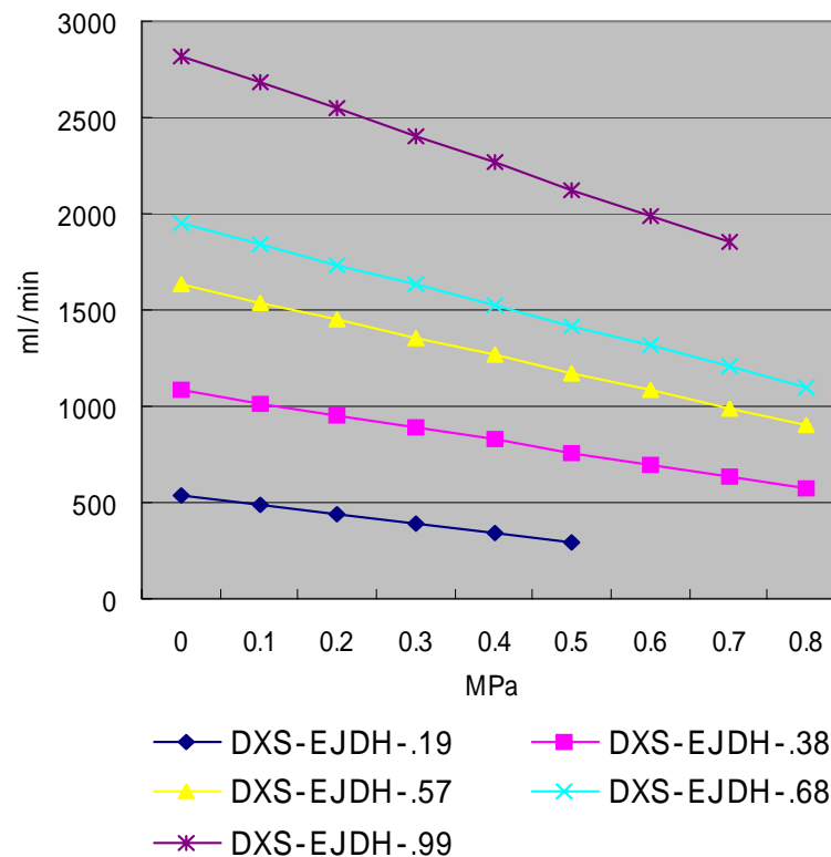
DXS-EJDH型 性能曲線
