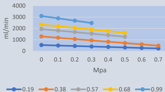
DDS-E015型性能曲線表
