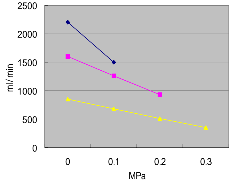
DDS-E034型 性能曲線
