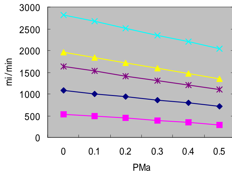
DDS-ED24型 性能曲線
