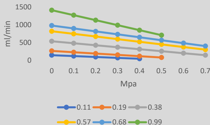
DDS-EJDC性能曲線
