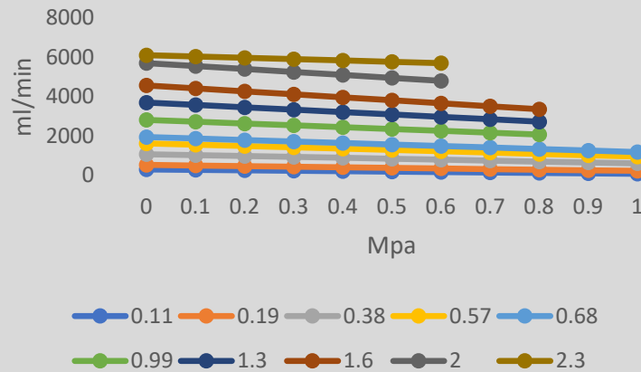
DXS-EBLE性能曲線
