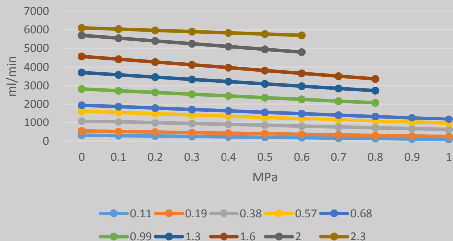
DXS-EJBE性能曲線
