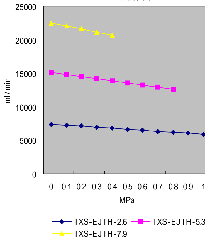
TXS-EJTH型 性能曲線
